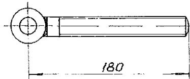
SKLOP ZAVRTNJA 2
