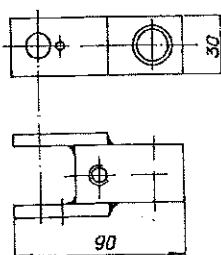
SKLOP VILJUŠKE 2
